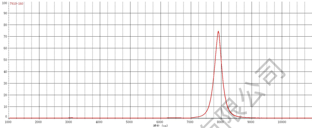
7.91um 红外窄带滤光片透射曲线图
