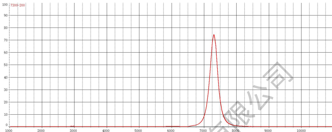
7. 30um 红外窄带滤光片透射曲线图
