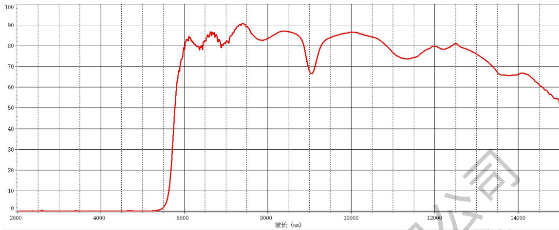
5500nm 红外长波通滤光片透射曲线图
